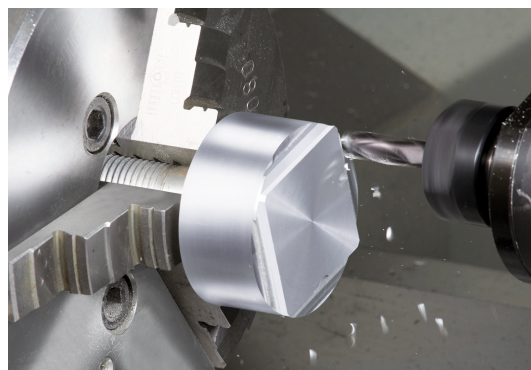
C-Achsenantrieb
